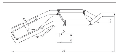
Typ N-2 a = max. 30 mm r = min. 1mm
