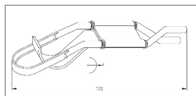
Typ N-1 r = max. 15 mm
