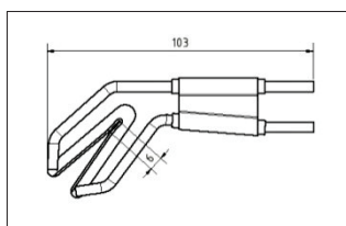
Typ HS-S-15° mit Schlitz und Anschlag
