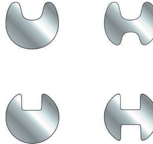
Vergleich herkömmliche Nadelgeometrie (untere Reihe) und LoopControl®-Geometrie (obere Reihe)
